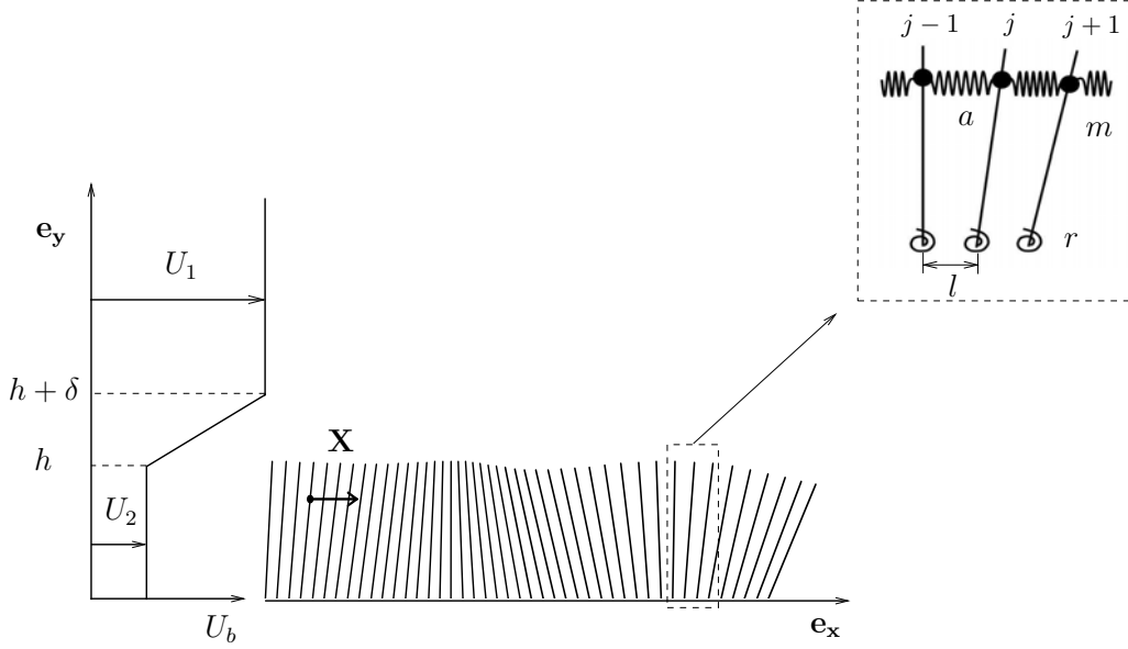
FIG. 3.1 – Représentation schématique du modèle couplé : profil de l'écoulement de base, U_b(y) , avec \delta l'épaisseur de vortacité, et modèle du couvert végétal où m , r et a sont respectivement la masse modale, la raideur en flexion et la raideur d'interaction.
