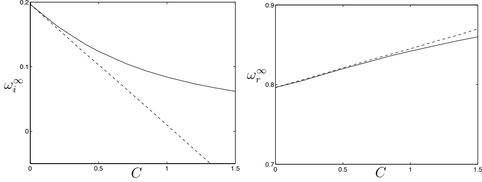
FIG. 3.12 – Taux de croissance et fréquence du modèle rigide en fonction du coefficient de couplage C : comparaison du résultat de l'analyse asymptotique (—) avec la solution exacte de (3.24) (—). L'évolution du nombre d'onde est équivalente à celle de la fréquence.
