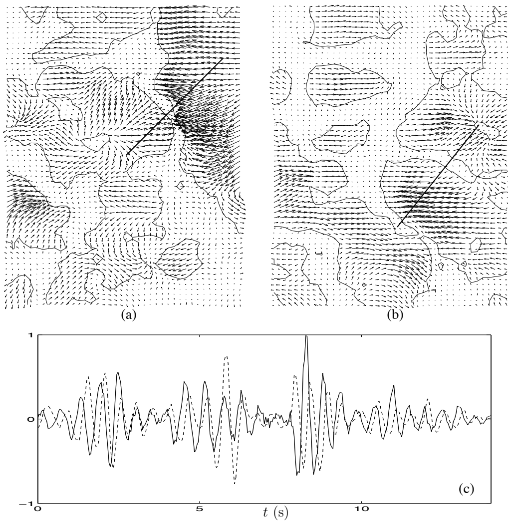
FIG. 2.10 – Illustration de la BOD sur une autre séquence de mouvement du champ de blé : topos 1 et 2 (a, b) avec superposition des iso-contours du module de vitesse, et chronos associés (c) : (—) chronos 1, (- -) chronos 2. La longueur d'onde \lambda (représentée par le trait) est ici environ 1.30 m pour les deux topos, et la fréquence f des chronos 1.85 Hz. Ces deux premiers modes représentent respectivement 13% et 8% de l'énergie totale.
