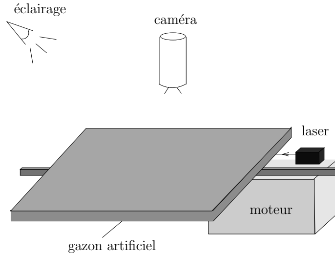
FIG. 2.3 – Schéma du montage visant à tester en laboratoire la technique de mesure du mouvement du couvert par PIV.
