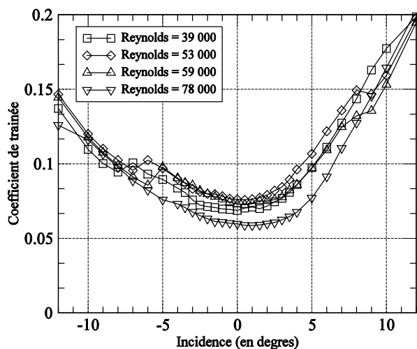
Figure 73. Coefficients de trainée ( C_D ) de la maquette du viaduc de Millau en fonction de l'incidence
