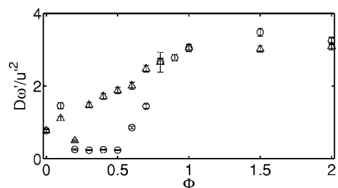
FIG. 6. One-particle diffusion coefficient. n=1 . ( \Delta ) Re=1400 ; ( \circ ) Re=7000 .
